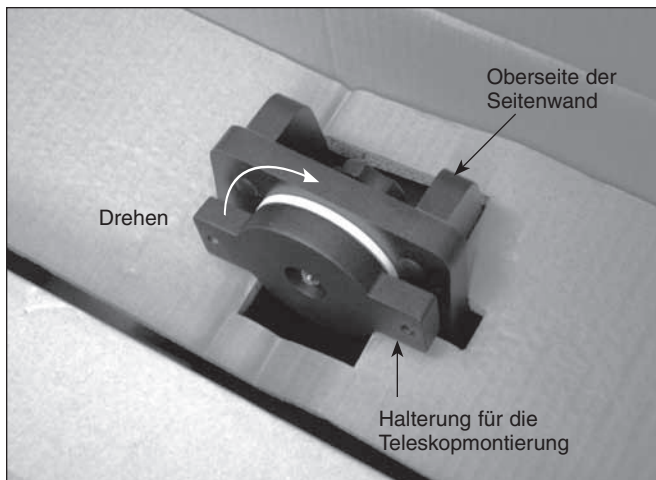
Abbildung 2. Um die Pappkartoneinlage an der Oberseite der azimutalen Montierung zu entfernen, drehen Sie die Halterung der Teleskopmontierung so, dass die Längsachse vertikal ausgerichtet ist. Entfernen Sie dann die Einlage.
