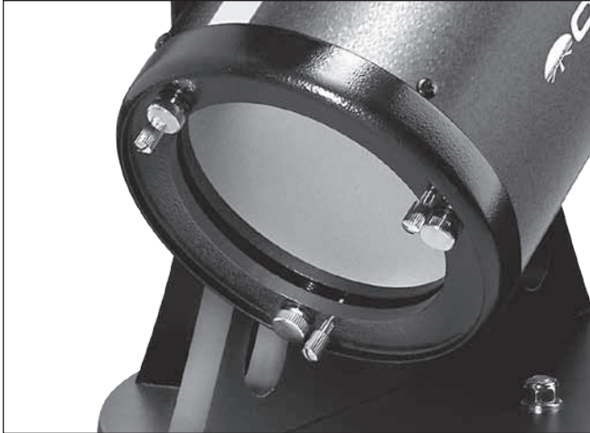
Abbildung 24. Die Rändelschrauben für Kollimation und Spiegelarretierung.
