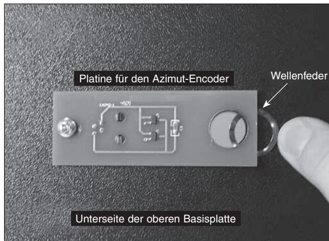
Abbildung 7. Die Wellenfeder wird zwischen der Platine für den Azimut-Encoder und der Basisplatte eingesetzt. Dabei muss die Aussparung der Wellenfeder an der Bohrung in der Mitte der Basisplatte ausgerichtet werden.
