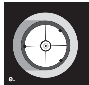
Abbildung 20. Kollimieren der Optik. (a) Wenn die Spiegel richtig ausgerichtet sind, sollte die Ansicht längs des Okularauszugs des Fokussierers so aussehen. (b) Das Bild könnte etwa so aussehen, wenn die Optik bei eingesetzter Kollimationskappe falsch ausgerichtet ist. (c) Hier ist der Sekundärspiegel unter dem Fokussierer zentriert, aber er muss justiert (gekippt) werden, sodass der Primärspiegel vollständig sichtbar wird. (d) Der Sekundärspiegel ist korrekt ausgerichtet, aber der Primärspiegel muss noch eingestellt werden. Wenn der Primärspiegel richtig ausgerichtet wurde, ist der „Punkt“ der Kollimationskappe zentriert (wie in (e)).
