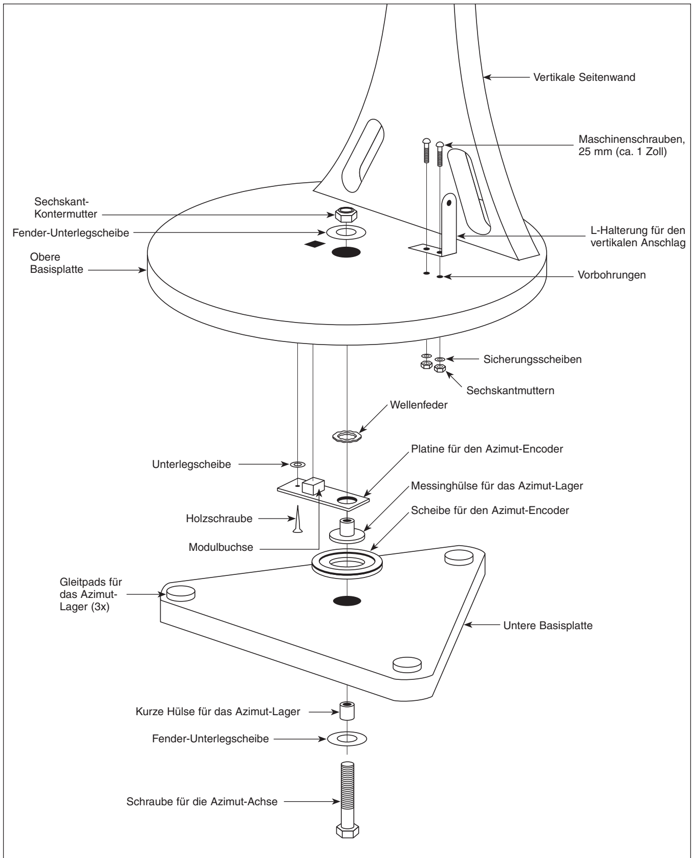
Abbildung 3. Diese Abbildung zeigt die korrekte Positionierung der Azimut-Komponenten des IntelliScope-Systems an der azimutalen Montierung.
